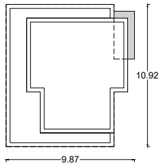
[PLANTA DE COBERTURA]
